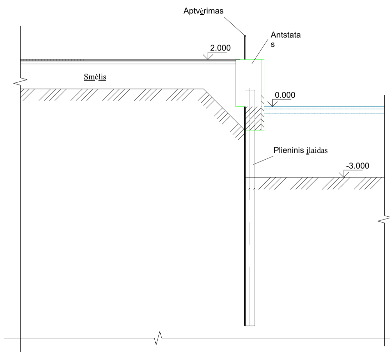
Krantinės pjūvis
