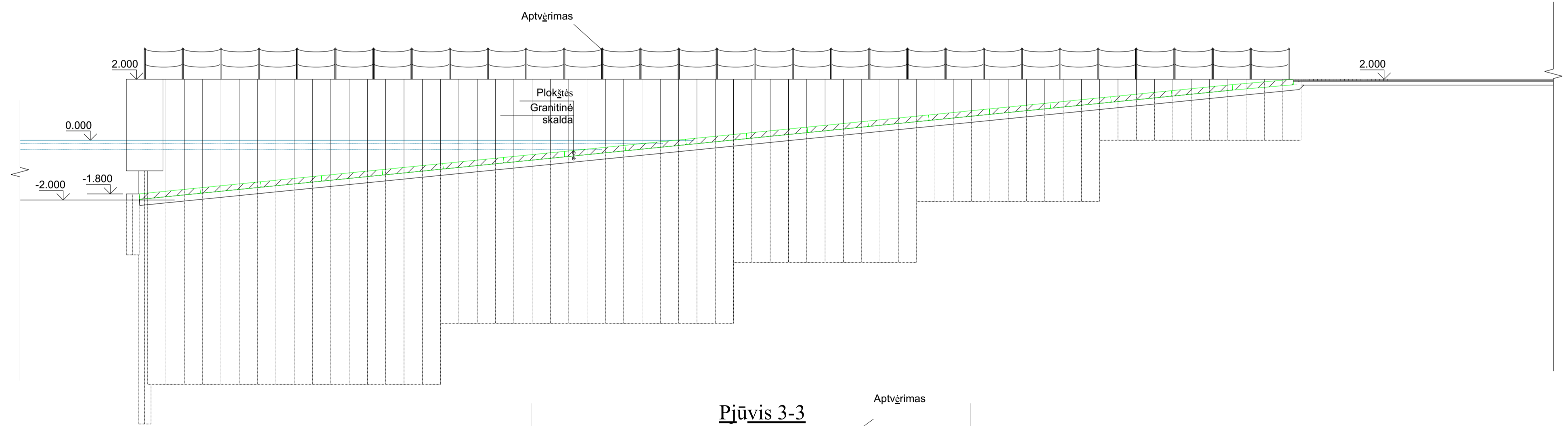
Slipo pjūvis
